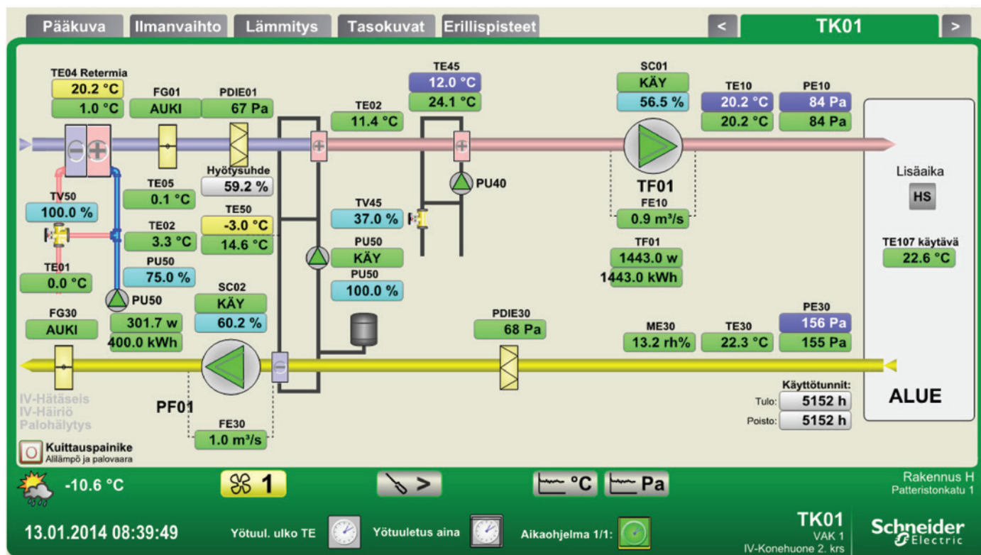
Valvomonäkymä MAMK H-rakennuksen passiivijärjestelmästä. Tuloilman lämpötila neulalämmönsiirtimen jälkeen on +1,0 °C ulkoilman ollessa -10,6 °C.
